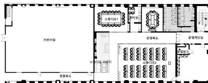
전시공간 도면
